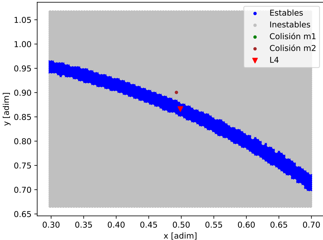
Mapa de estabilidad - Kepler-42_Kepler-42_c
