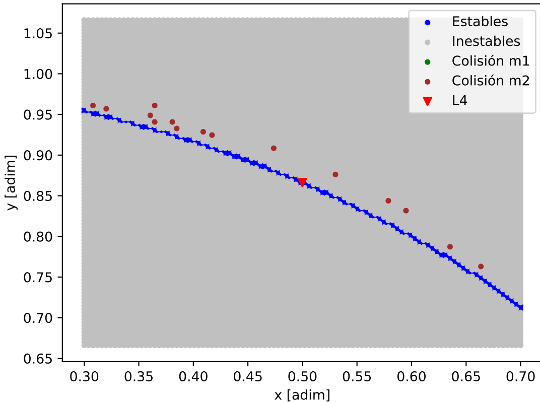
Mapa de estabilidad - Kepler-445_Kepler-445_b
