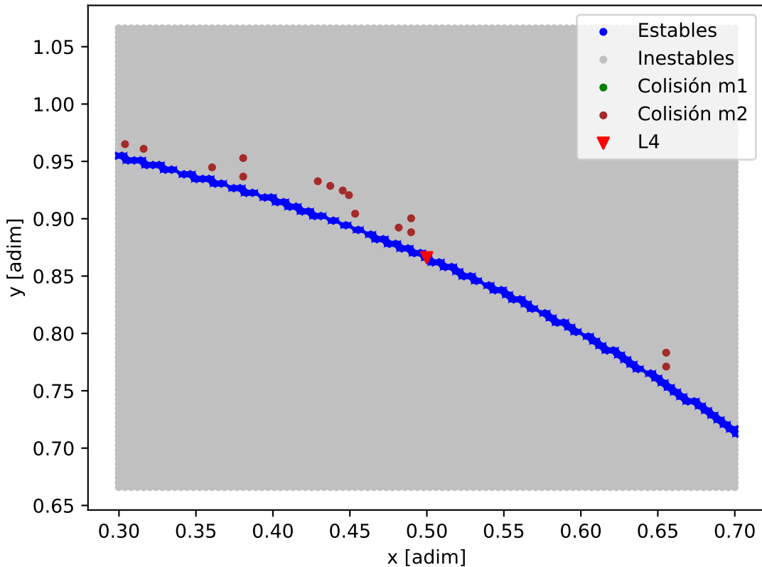
Mapa de estabilidad - Kepler-445_Kepler-445_c
