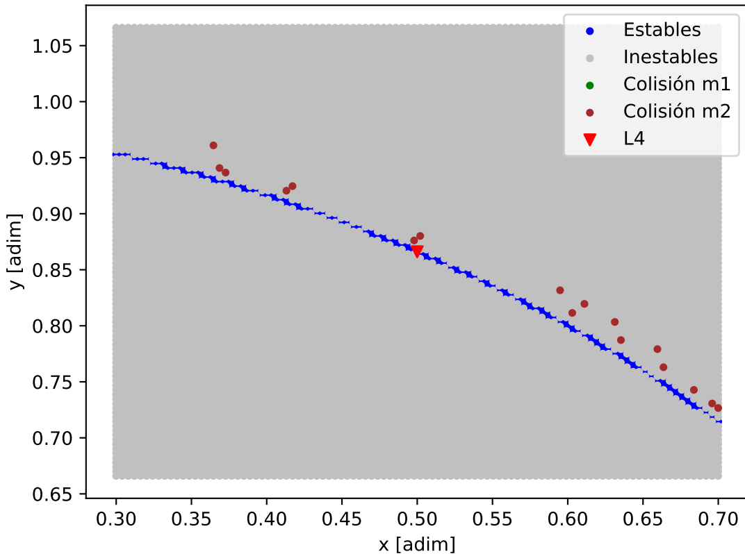
Mapa de estabilidad - Kepler-445_Kepler-445_d
