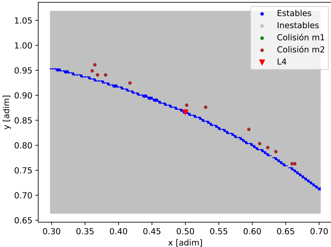
Mapa de estabilidad - Kepler-49_Kepler-49_b
