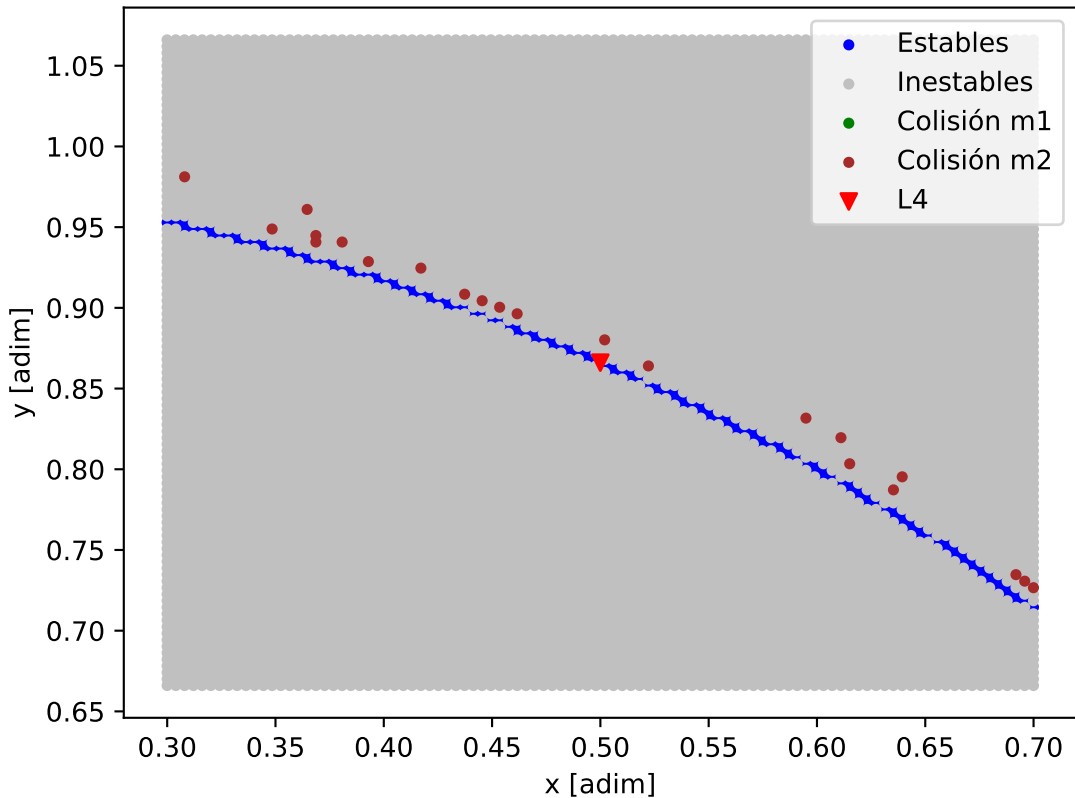
Mapa de estabilidad - Kepler-49_Kepler-49_c
