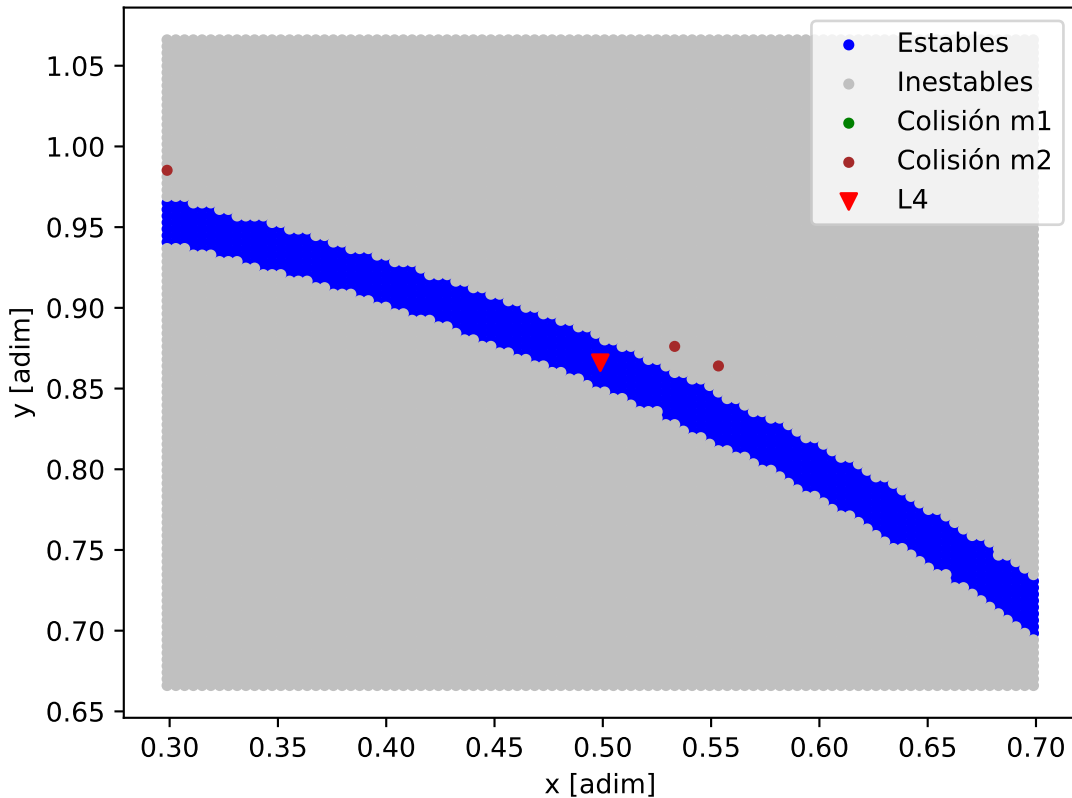
Mapa de estabilidad - Kepler-49_Kepler-49_d
