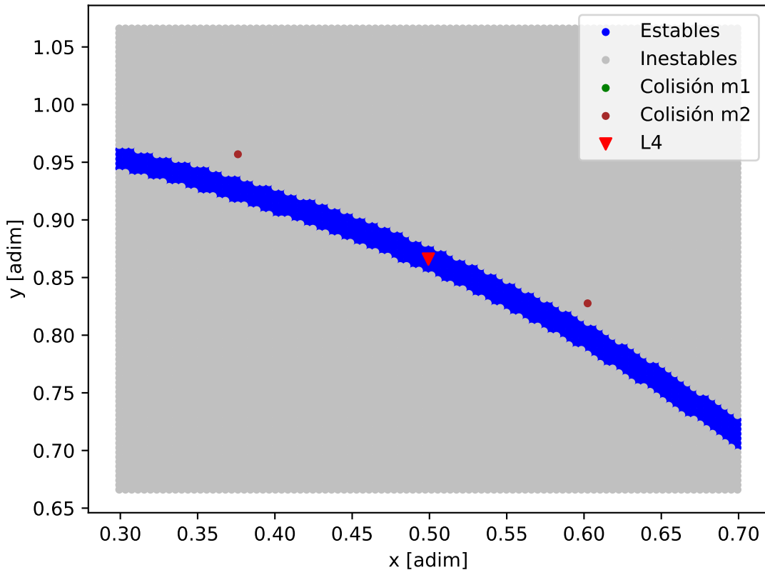
Mapa de estabilidad - Kepler-52_Kepler-52_b
