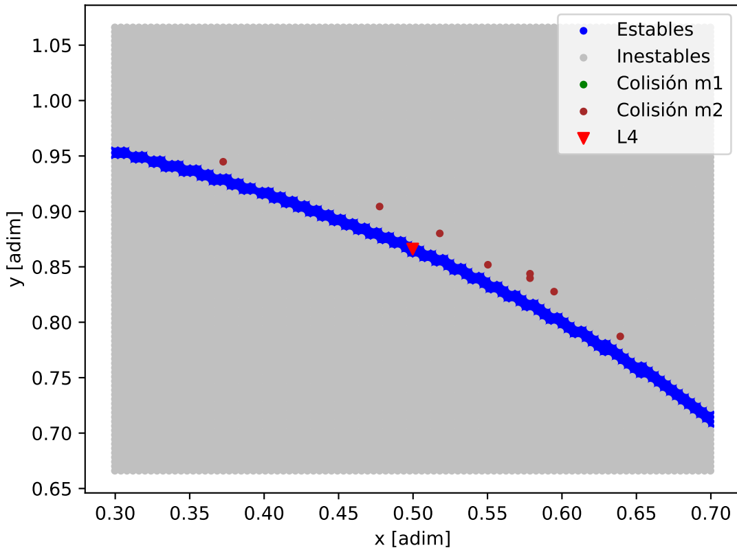
Mapa de estabilidad - Kepler-52_Kepler-52_c
