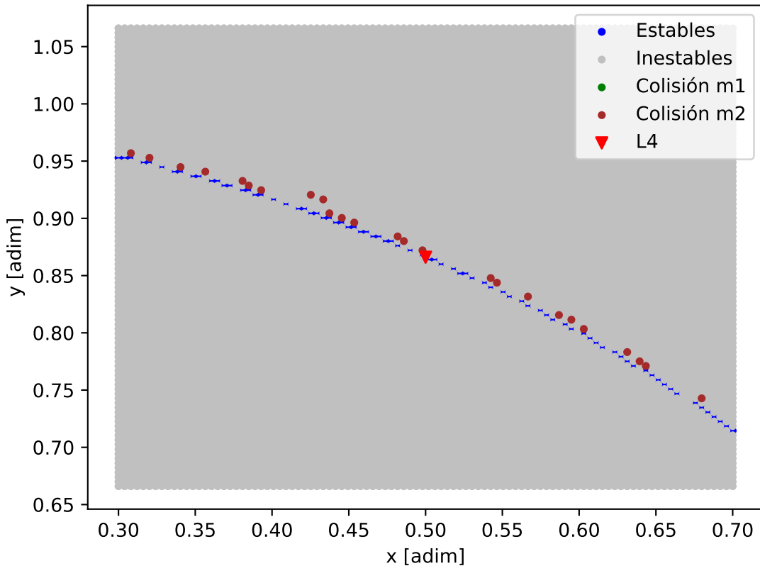
Mapa de estabilidad - Kepler-54_Kepler-54_b
