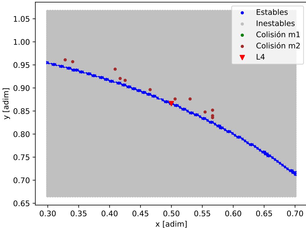
Mapa de estabilidad - Kepler-54_Kepler-54_d
