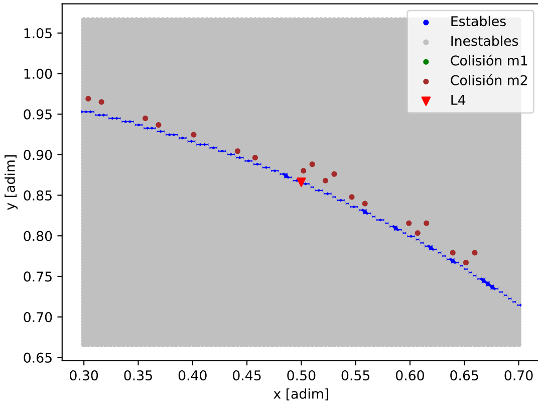
Mapa de estabilidad - Kepler-81_Kepler-81_c
