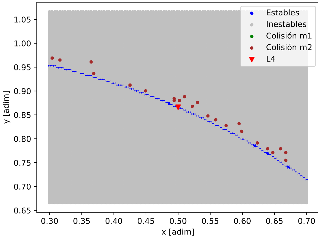
Mapa de estabilidad - Kepler-83_Kepler-83_d
