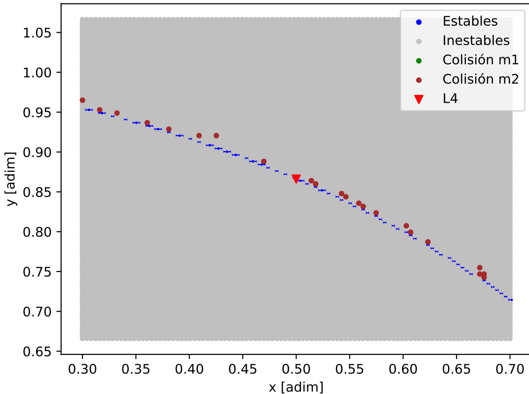
Mapa de estabilidad - LHS_1678_LHS_1678_b
