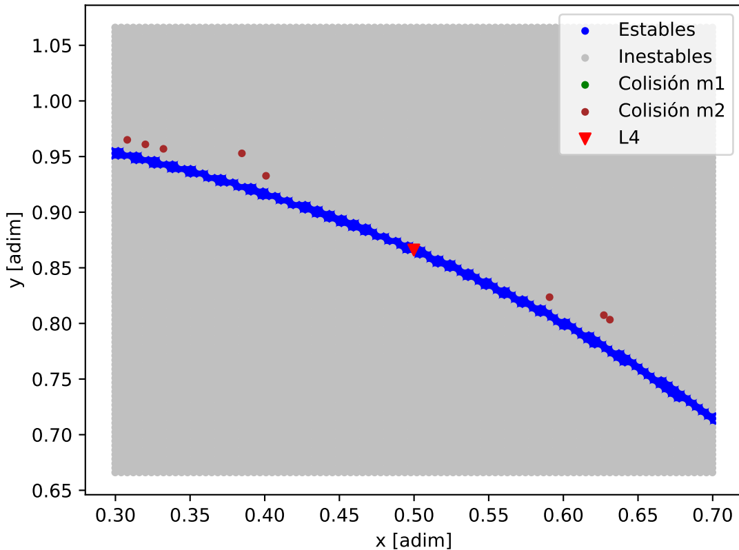
Mapa de estabilidad - LP_791-18_LP_791-18_c
