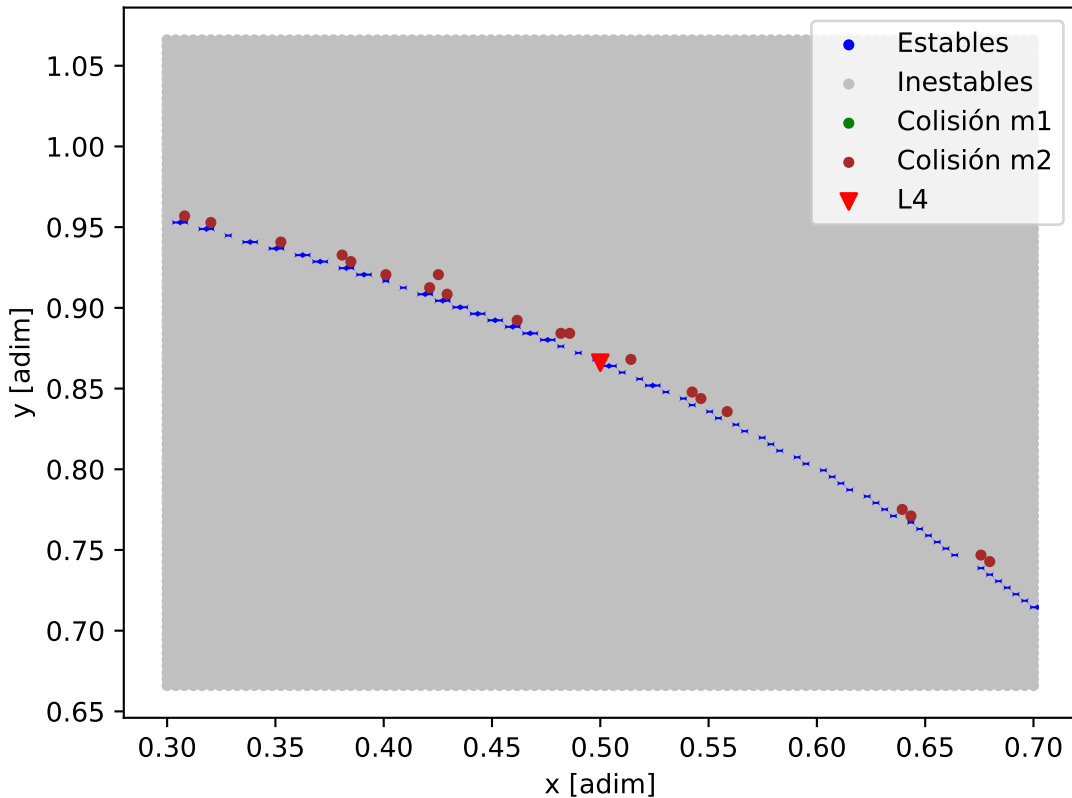
Mapa de estabilidad - L_98-59_L_98-59_b
