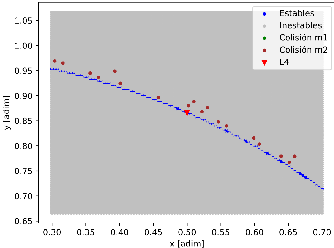
Mapa de estabilidad - L_98-59_L_98-59_c
