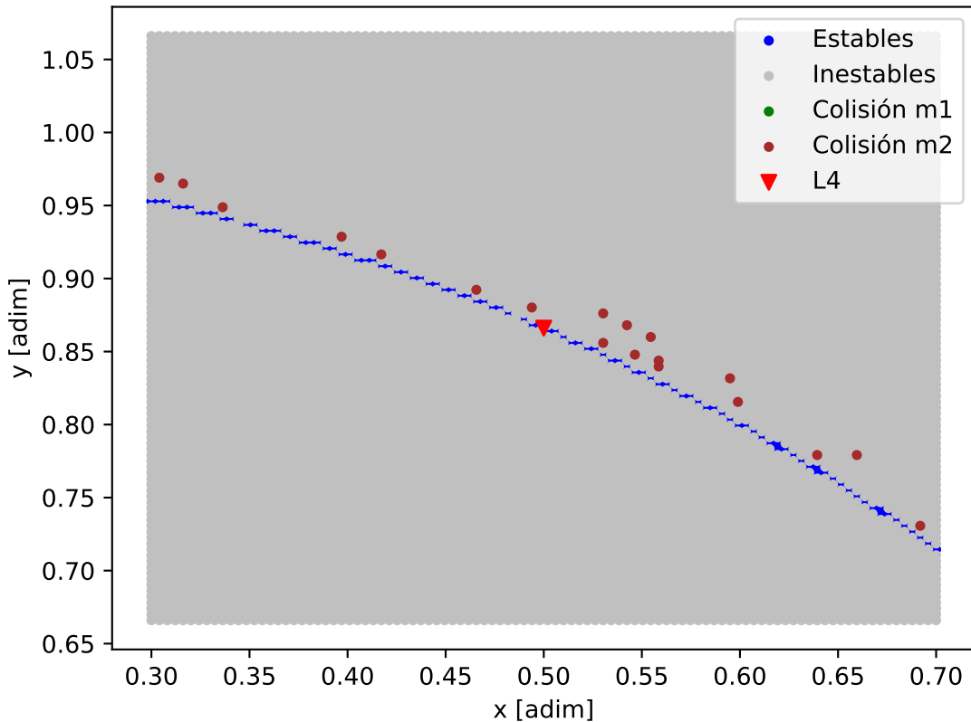
Mapa de estabilidad - L_98-59_L_98-59_d
