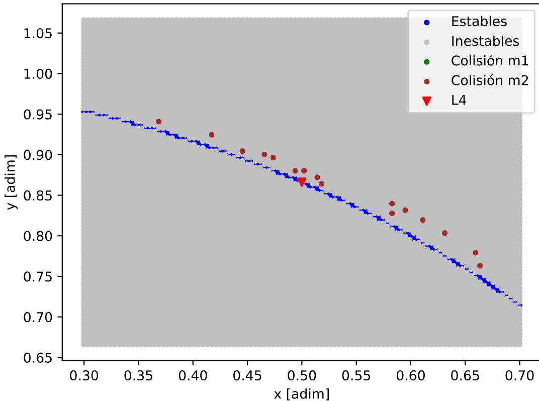
Mapa de estabilidad - TOI-1266_TOI-1266_b
