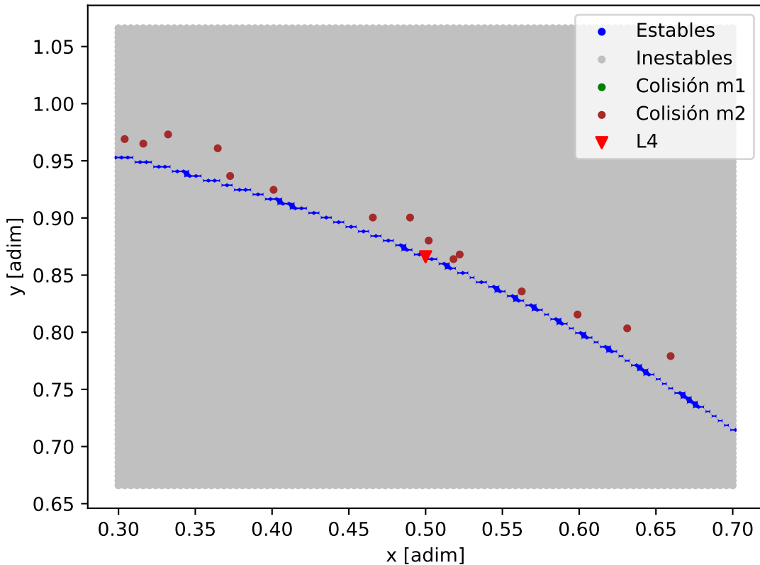
Mapa de estabilidad - TOI-1266_TOI-1266_d
