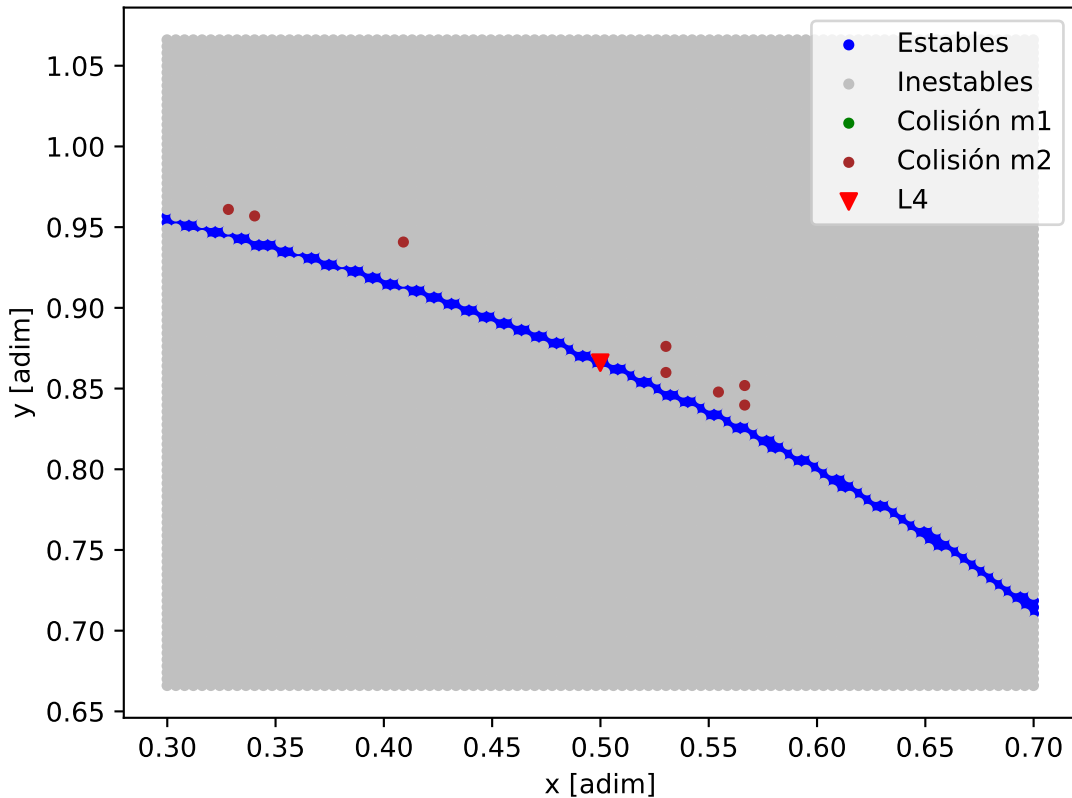
Mapa de estabilidad - TOI-1749_TOI-1749_c
