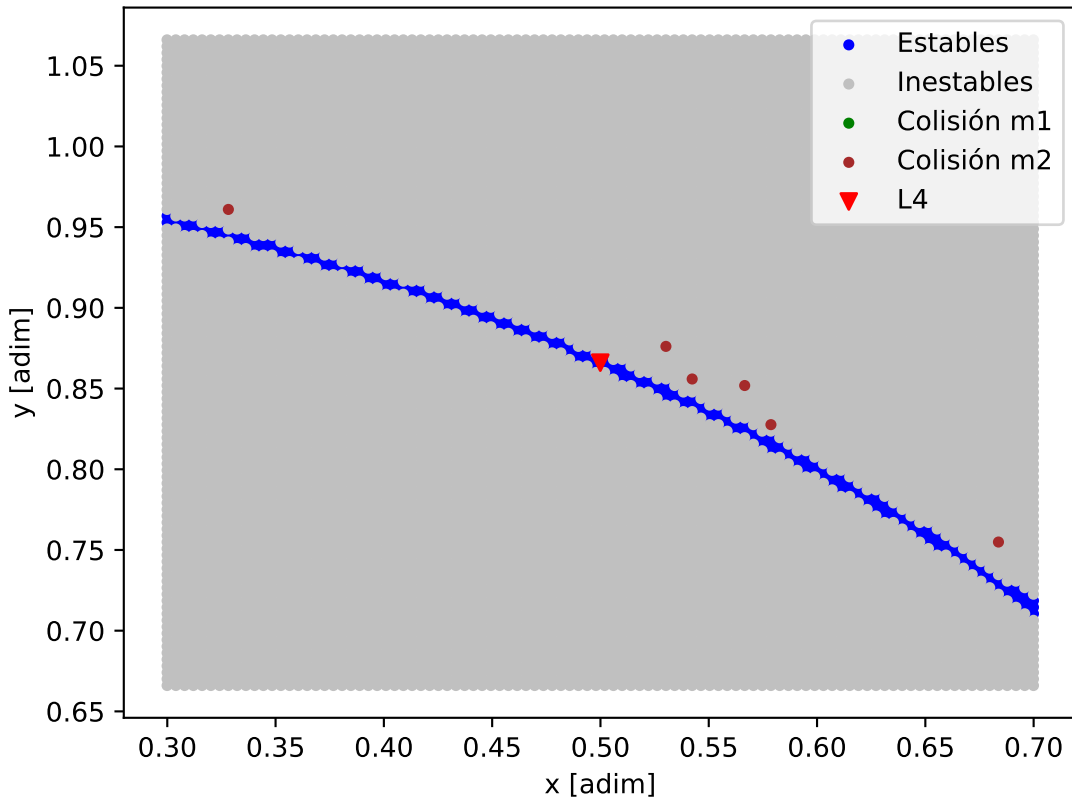
Mapa de estabilidad - TOI-1749_TOI-1749_d
