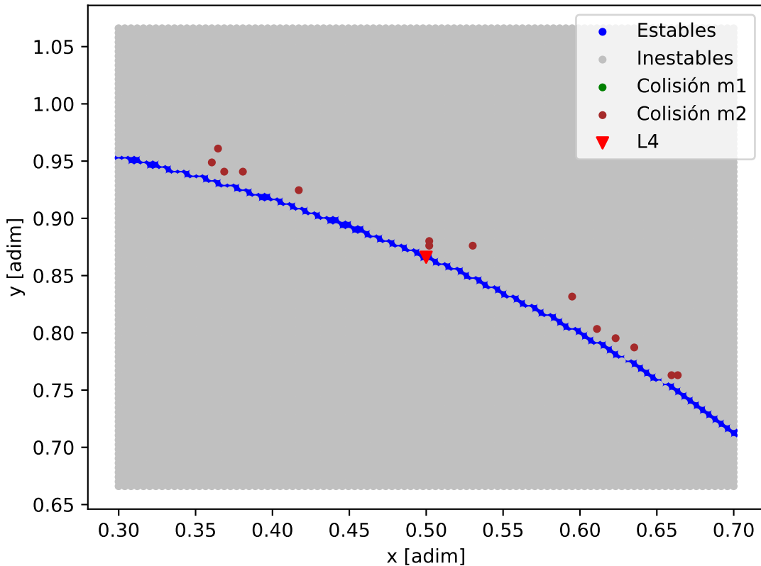
Mapa de estabilidad - TOI-270_TOI-270_c
