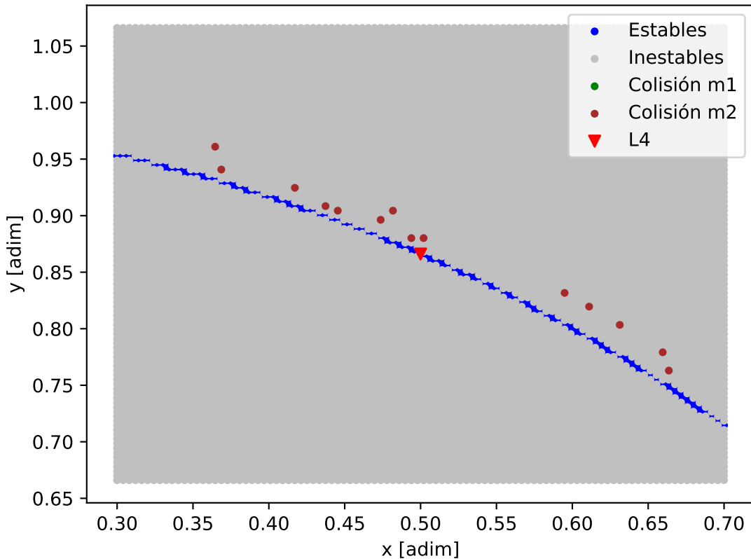
Mapa de estabilidad - TOI-270_TOI-270_d
