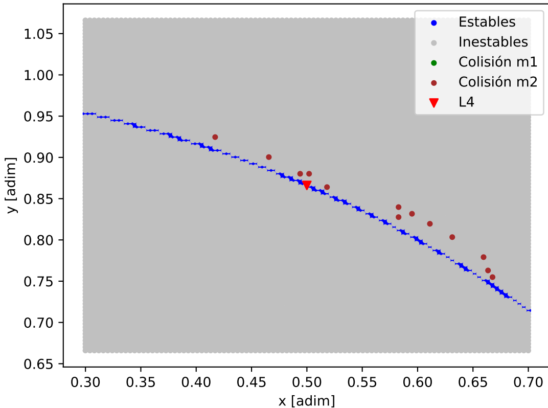
Mapa de estabilidad - TOI-663_TOI-663_d
