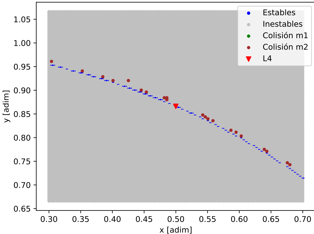
Mapa de estabilidad - TOI-700_TOI-700_b
