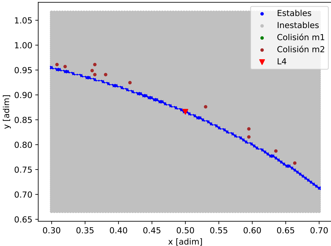
Mapa de estabilidad - TOI-700_TOI-700_c
