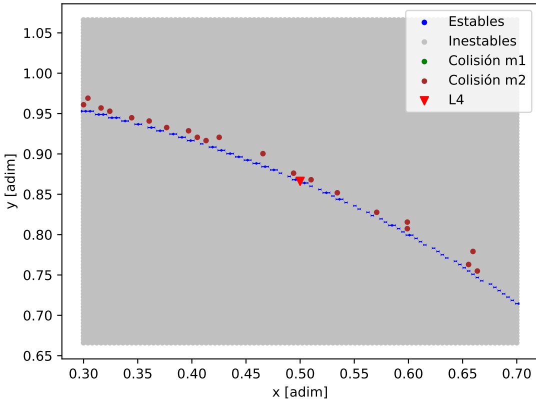
Mapa de estabilidad - TOI-700_TOI-700_d
