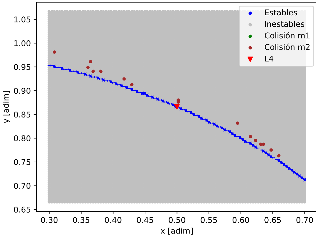
Mapa de estabilidad - TRAPPIST-1_TRAPPIST-1_b
