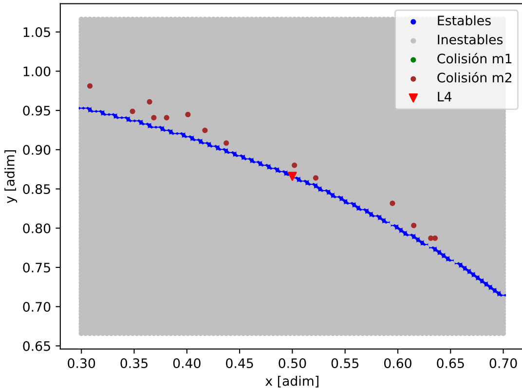
Mapa de estabilidad - TRAPPIST-1_TRAPPIST-1_c
