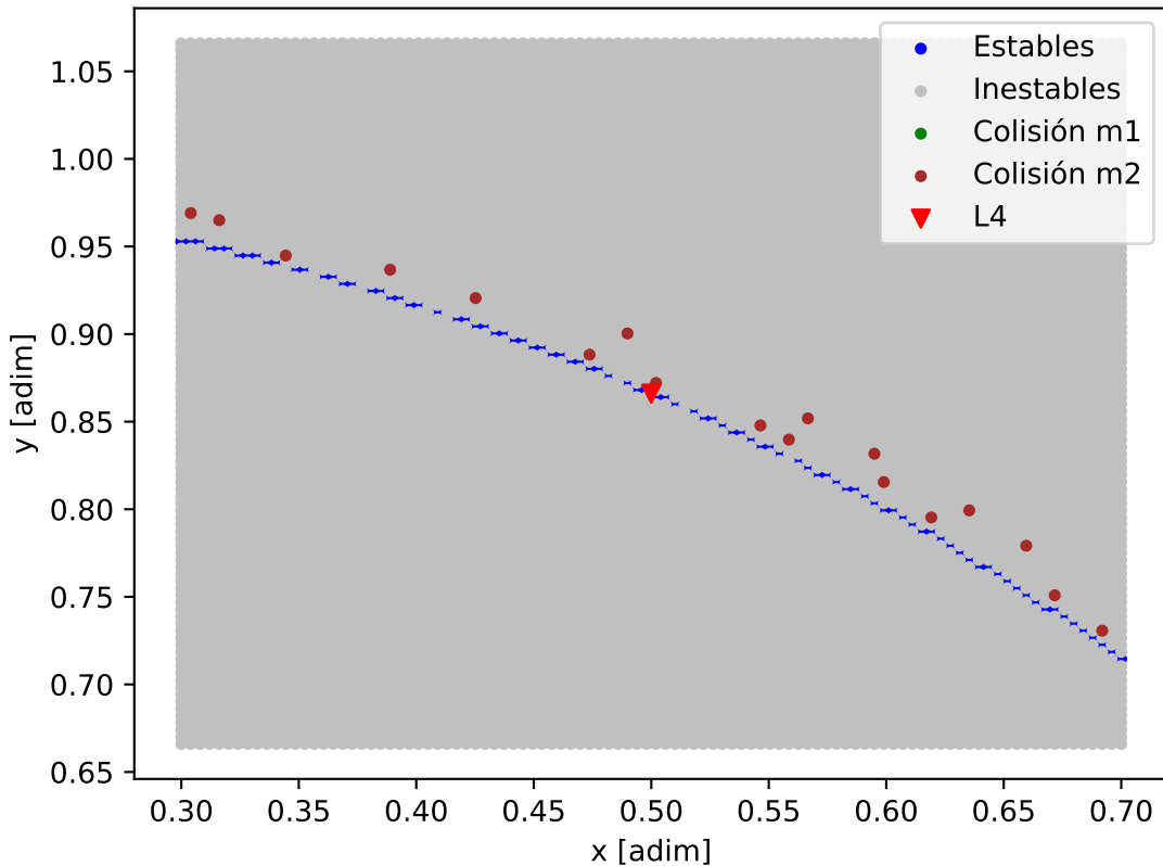
Mapa de estabilidad - TRAPPIST-1_TRAPPIST-1_d
