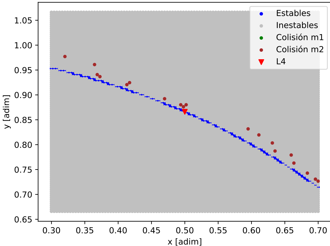
Mapa de estabilidad - TRAPPIST-1_TRAPPIST-1_f
