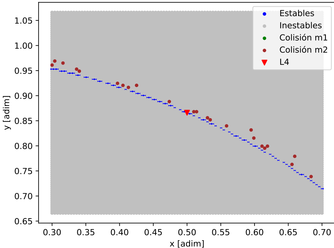
Mapa de estabilidad - TRAPPIST-1_TRAPPIST-1_h
