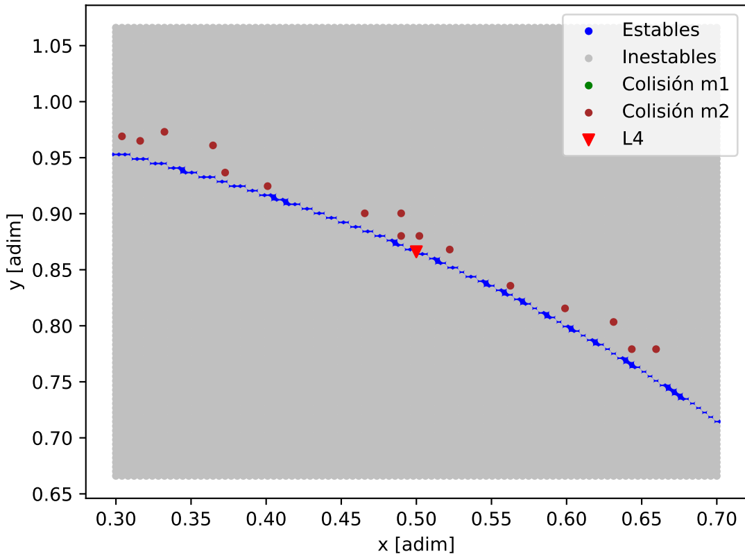
Mapa de estabilidad - Teegarden's_Star_Teegarden's_Star_d
