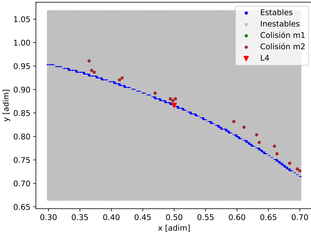
Mapa de estabilidad - Wolf_1061_Wolf_1061_c
