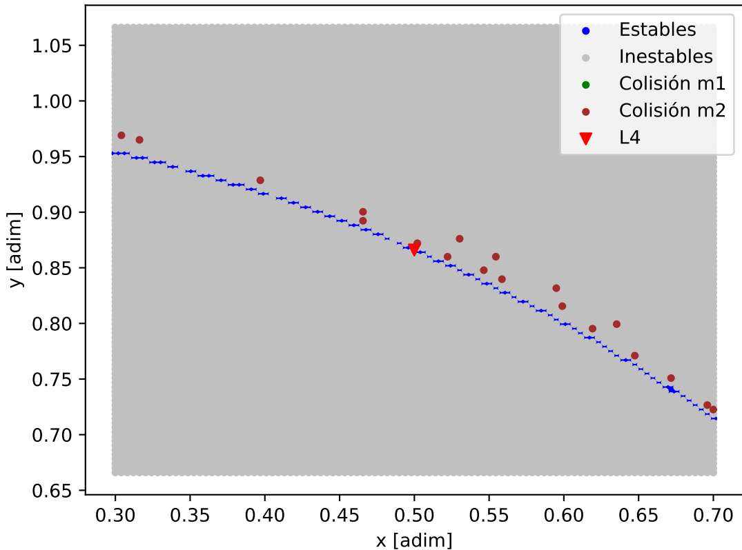
Mapa de estabilidad - YZ_Cet_YZ_Cet_b
