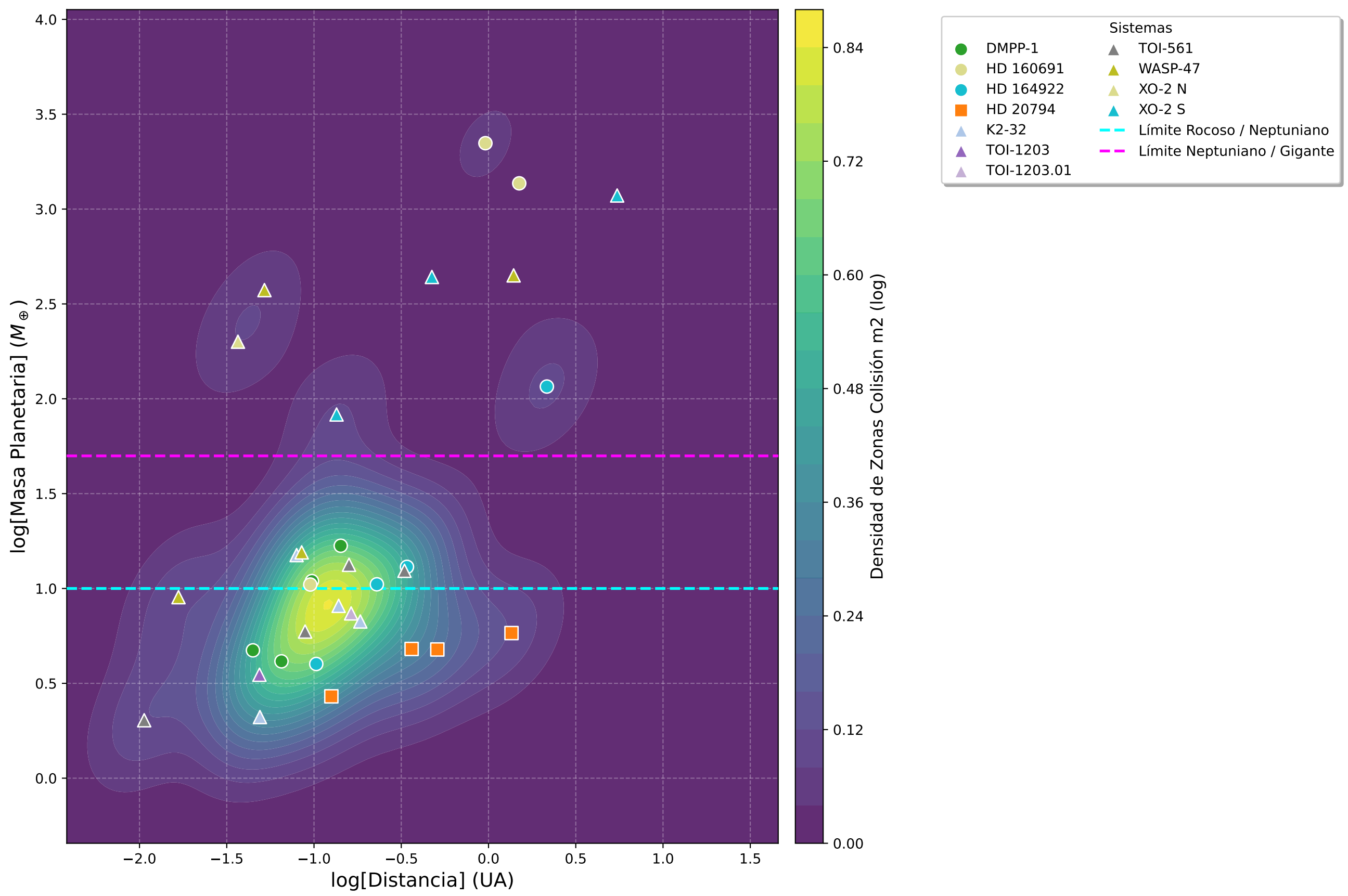
Sistemas con 5 planetas (Zonas Colisión m2)
