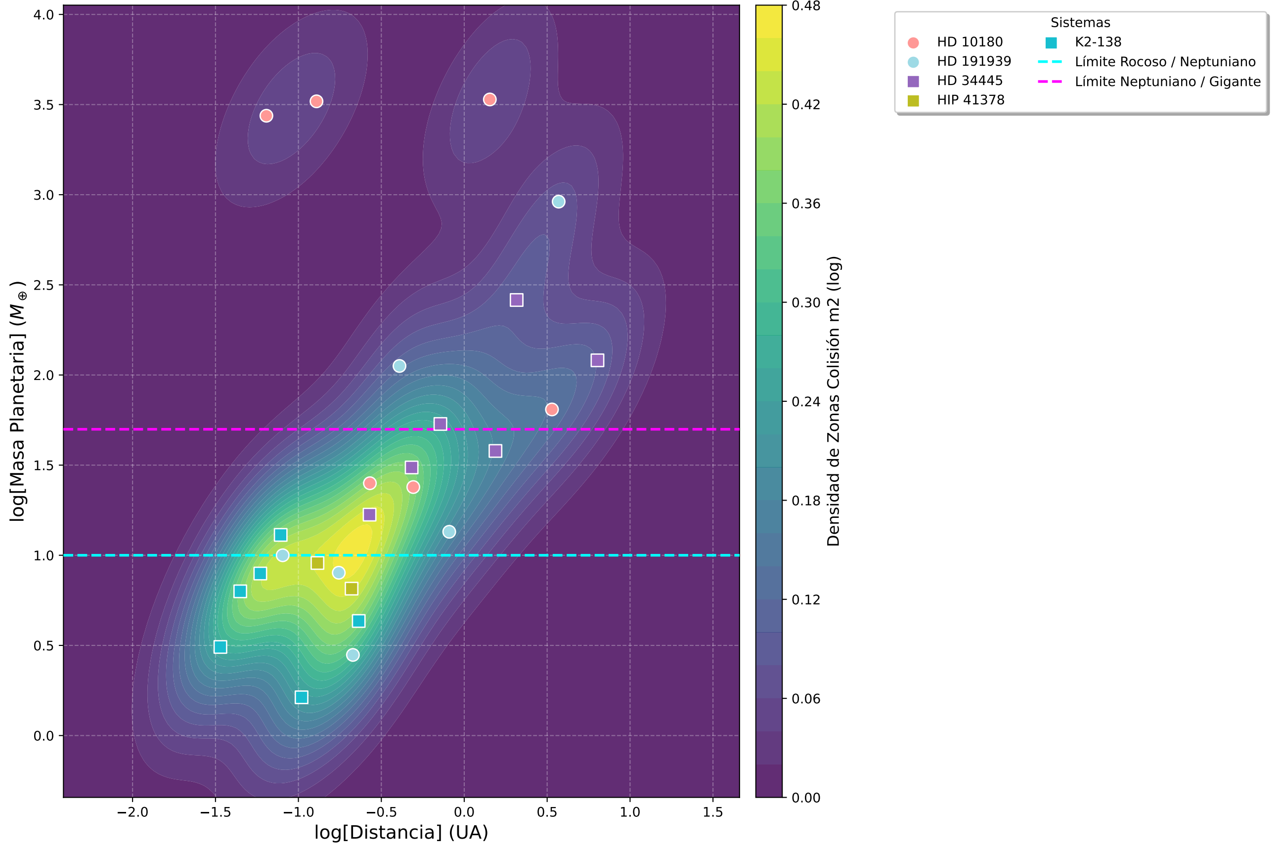
Sistemas con 7 planetas (Zonas Colisión m2)
