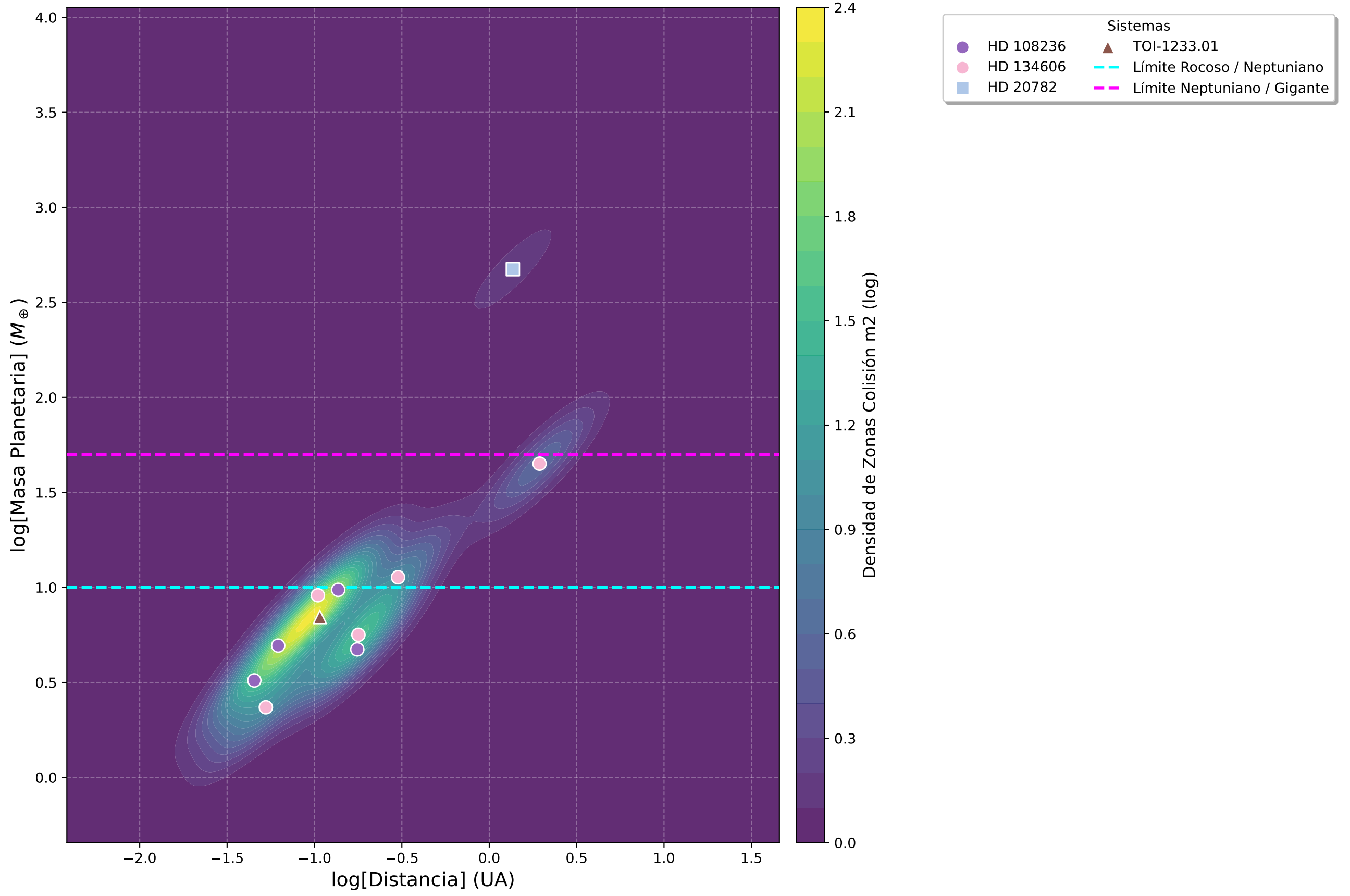
Sistemas con 6 planetas (Zonas Colisión m2)
