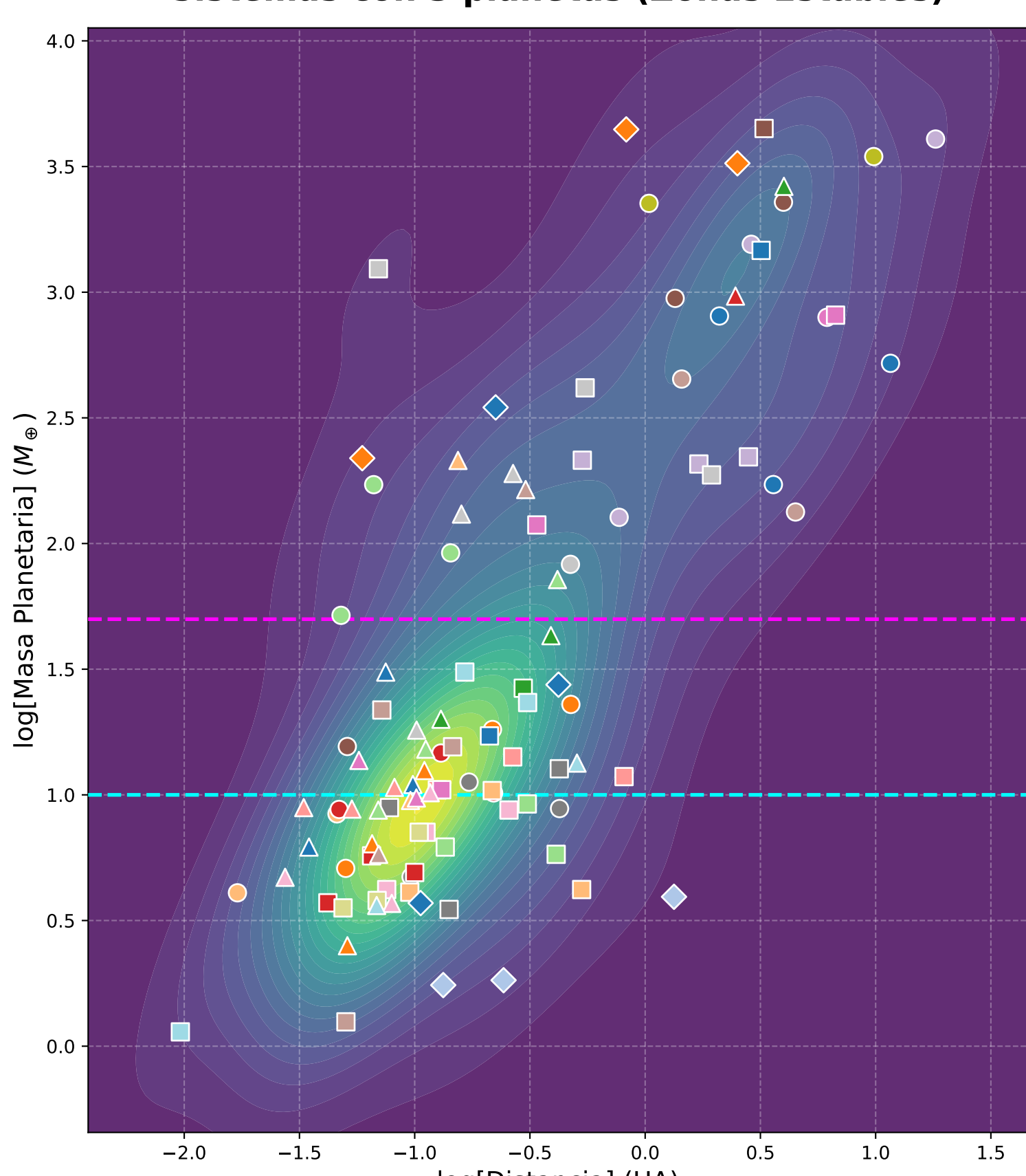
Sistemas con 4 planetas (Zonas Estables)
