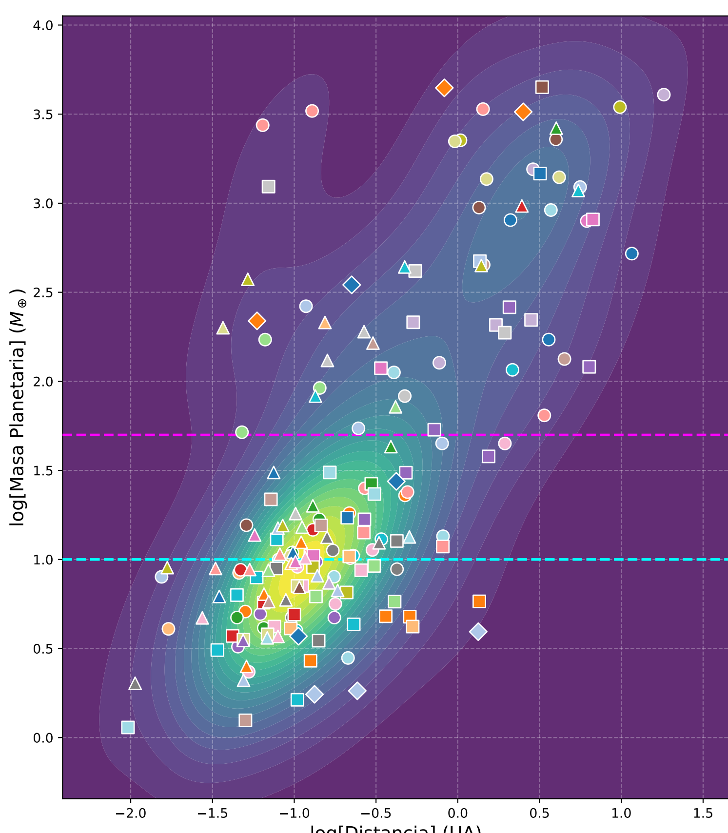
Sistemas con 3 planetas (Zonas Estables)
