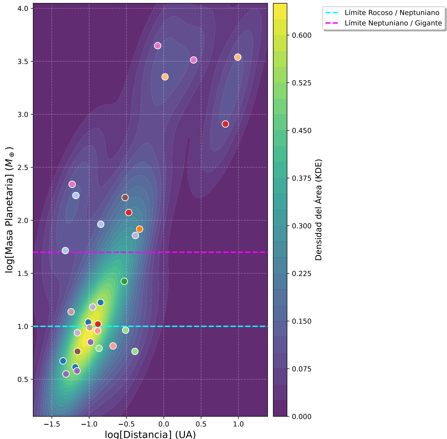
Sistemas con 3 planetas
