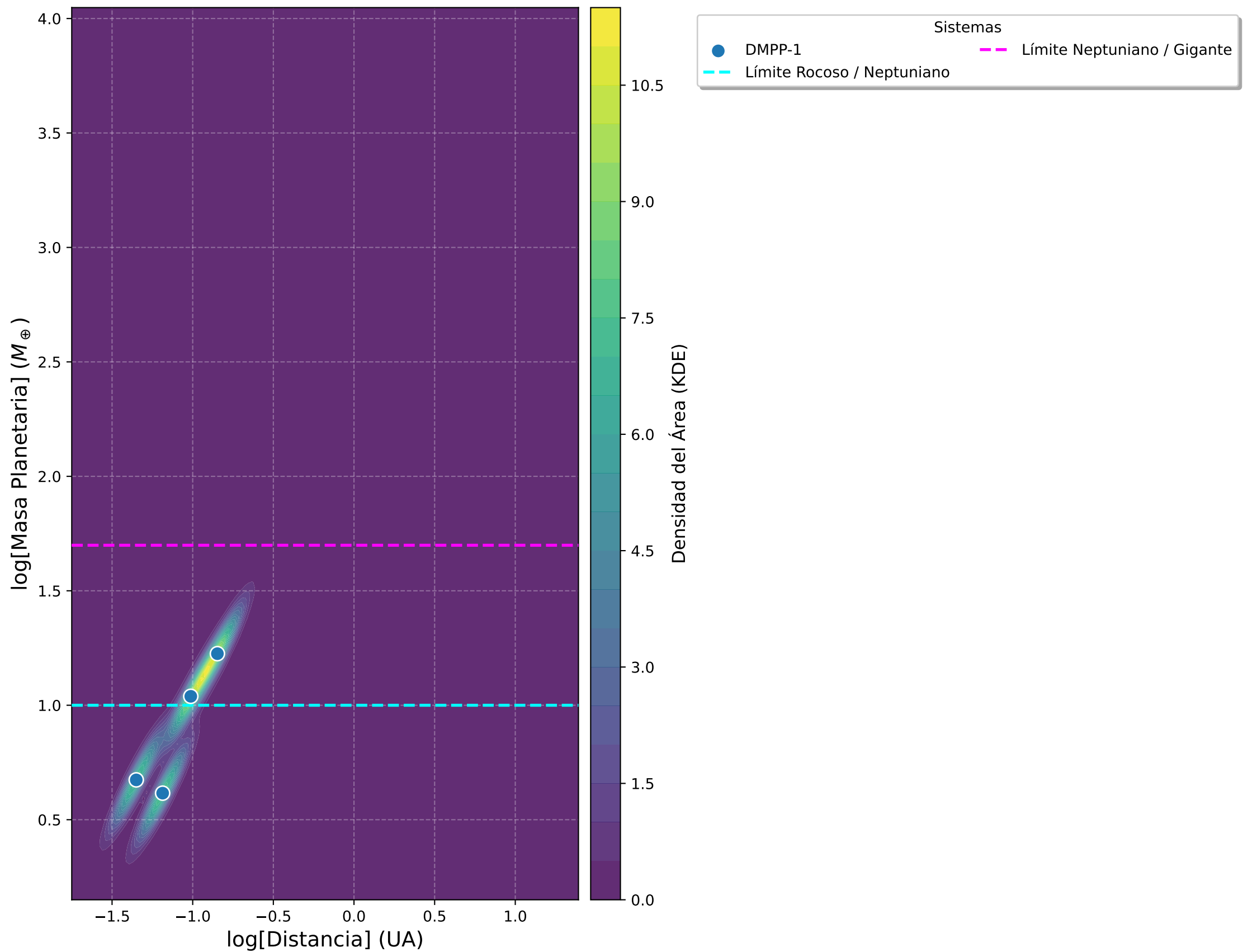
Sistemas con 6 planetas
