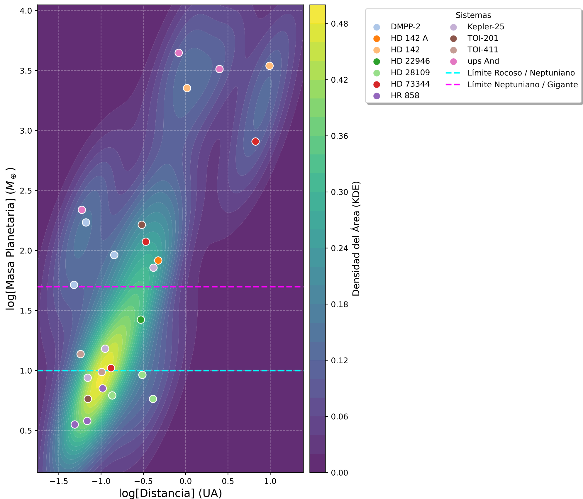
Sistemas con 4 planetas
