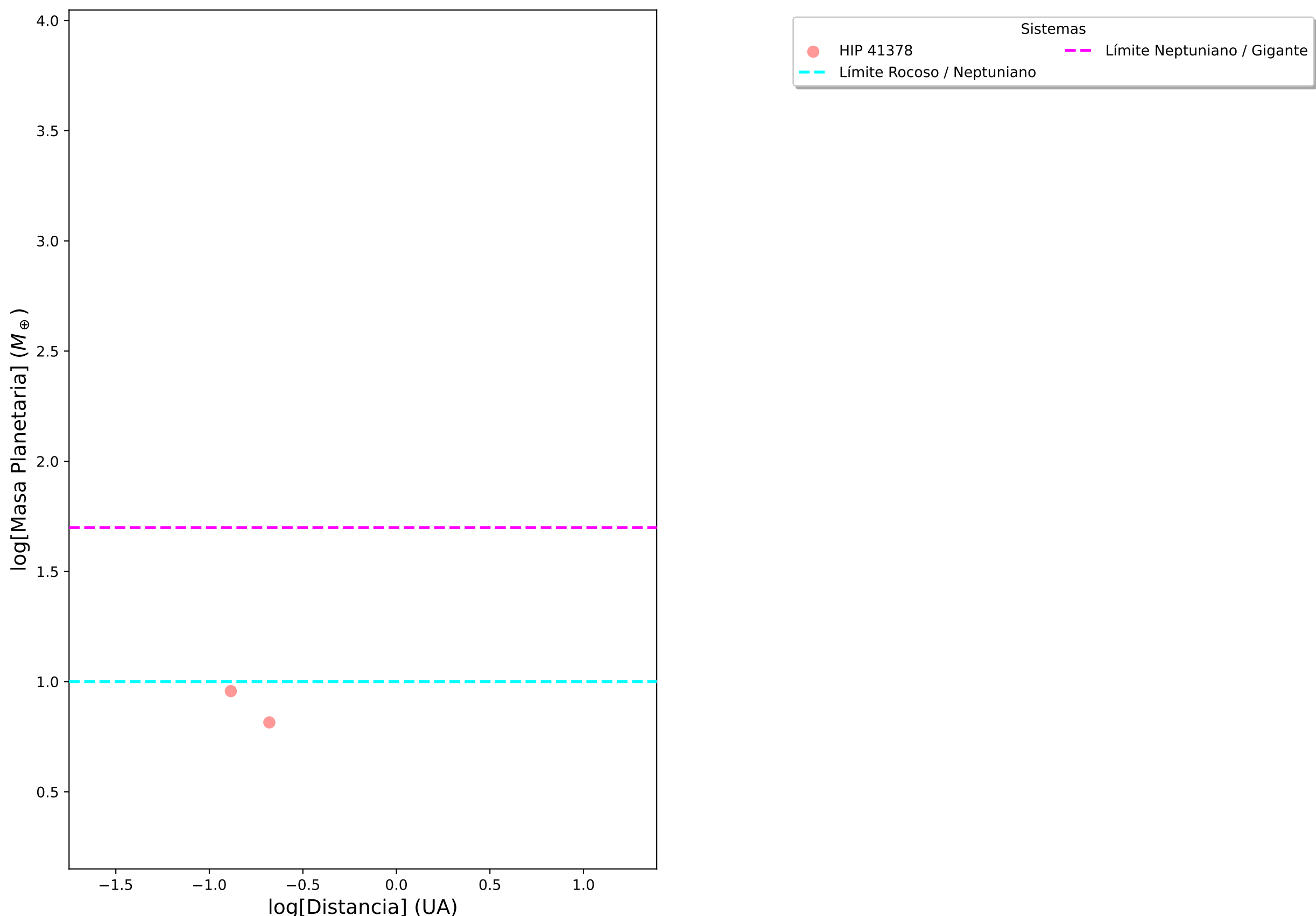
Sistemas con 6 planetas
