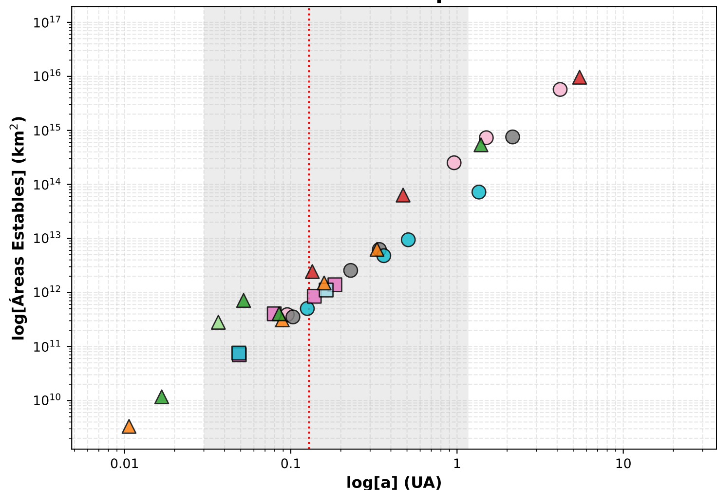
Sistemas con 5 planetas
