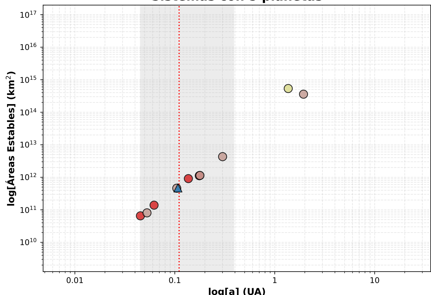
Sistemas con 6 planetas
