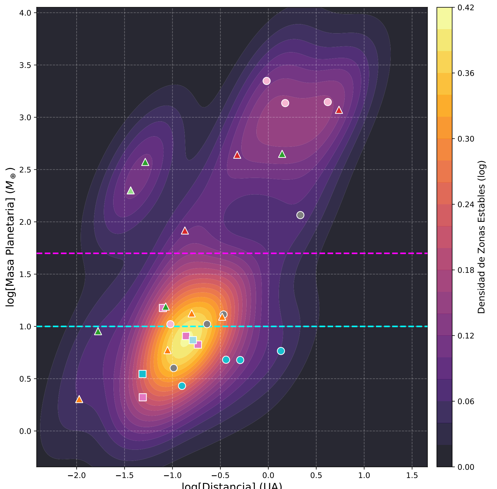
Sistemas con 5 planetas (Zonas Estables)
