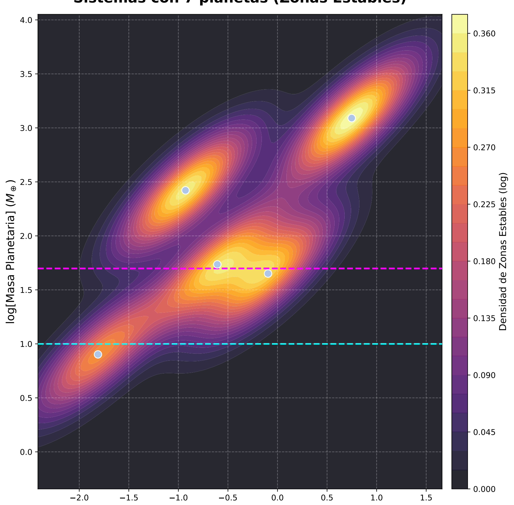
Sistemas con 7 planetas (Zonas Estables)
