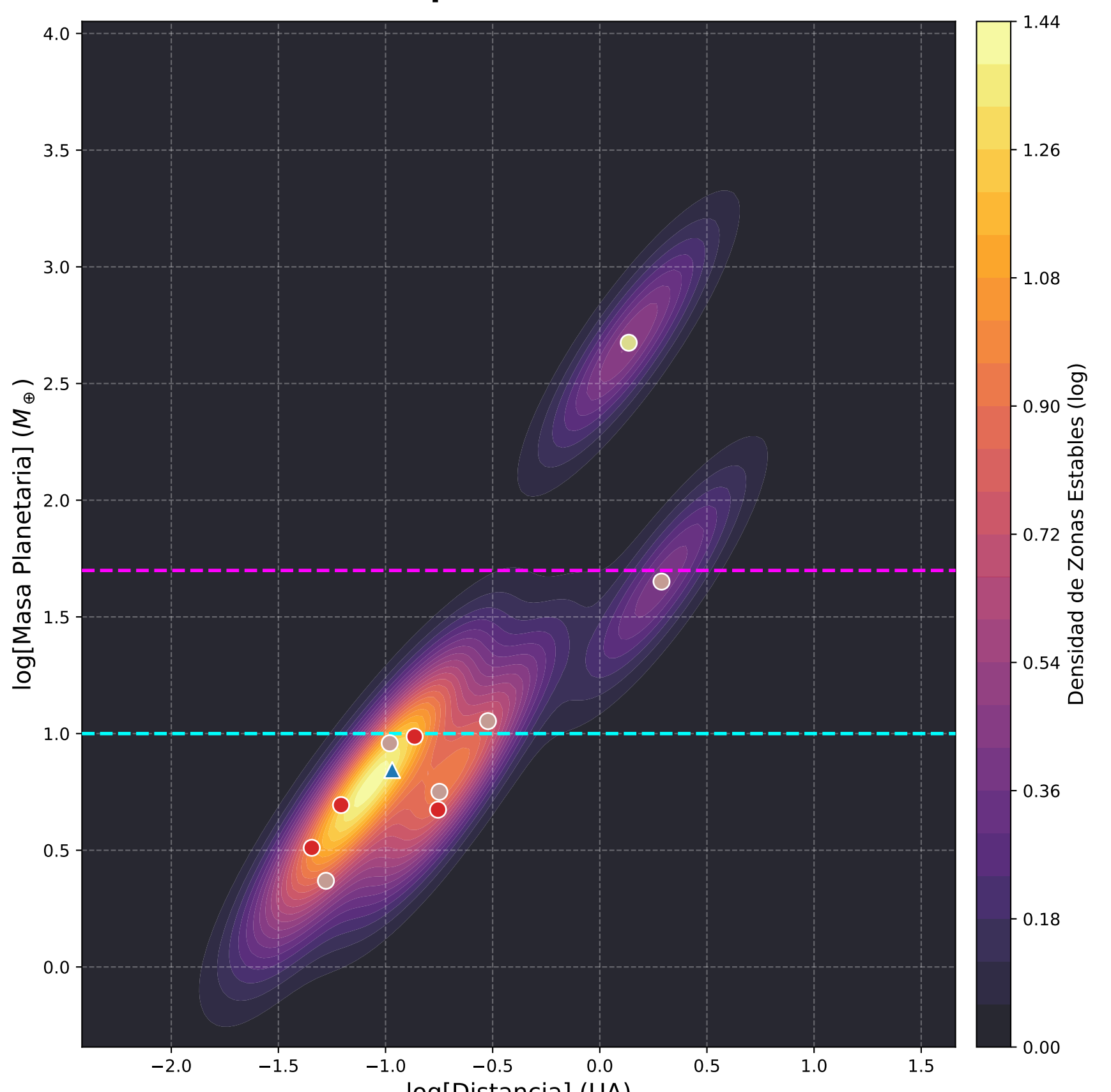
Sistemas con 6 planetas (Zonas Estables)
