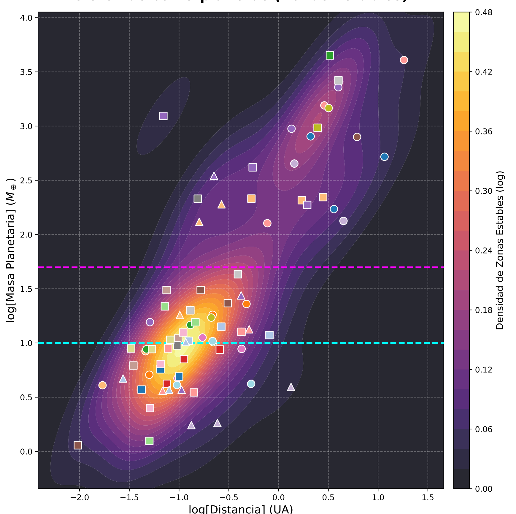
Sistemas con 4 planetas (Zonas Estables)
