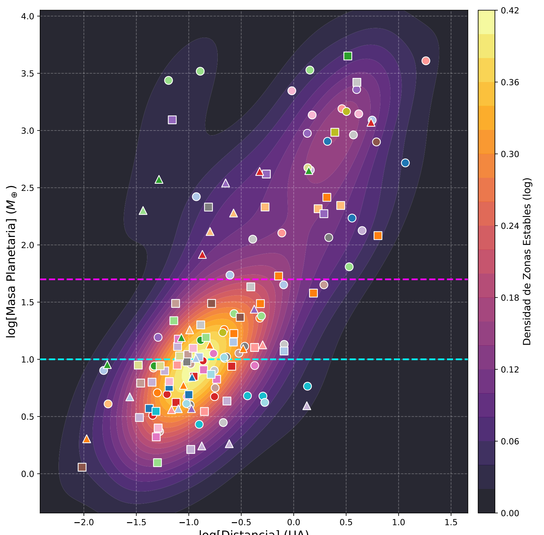
Sistemas con 3 planetas (Zonas Estables)
