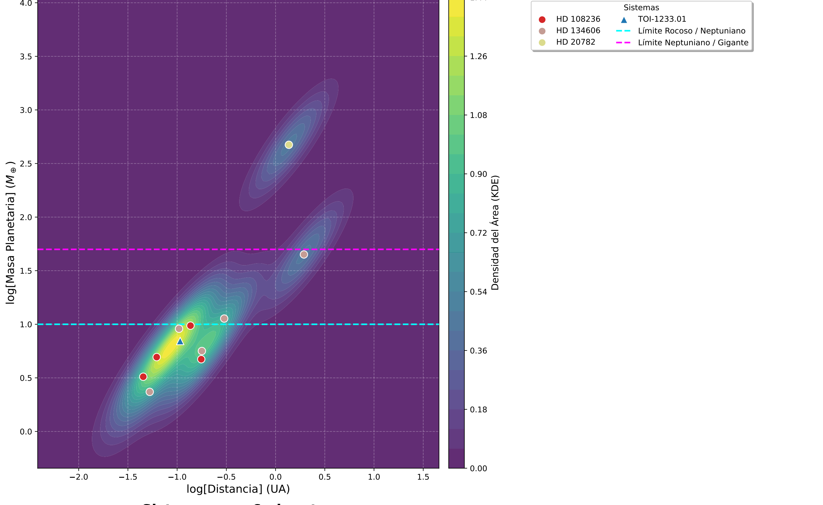
Sistemas con 6 planetas
