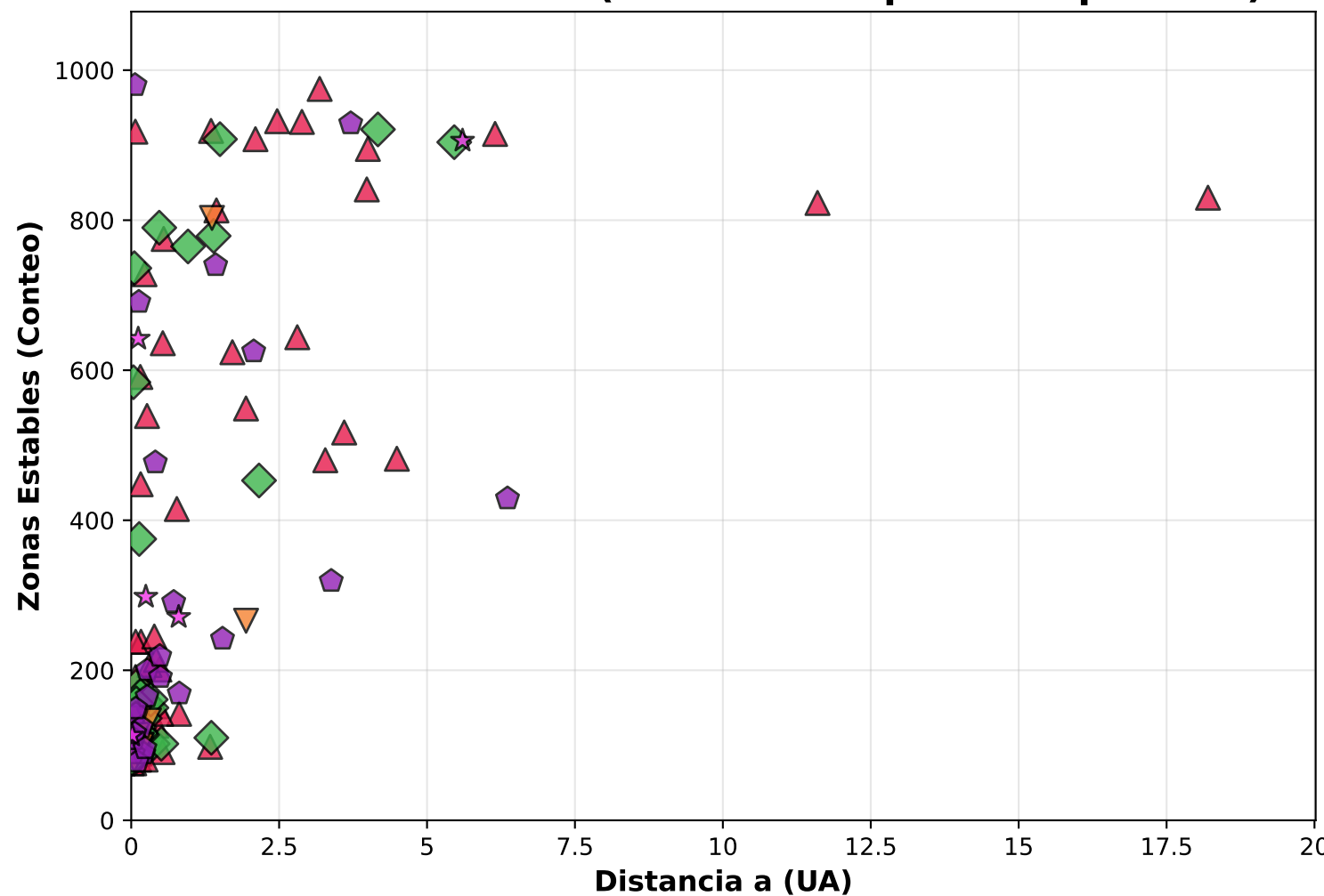
Sistemas con 3 planetas
