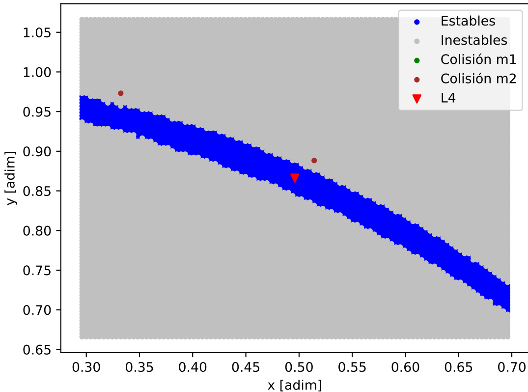
Mapa de estabilidad - HR_8799_HR_8799_b
