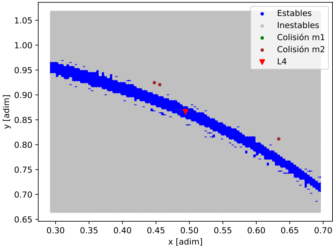
Mapa de estabilidad - HR_8799_HR_8799_d
