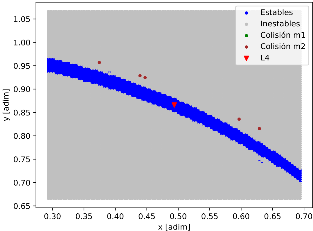
Mapa de estabilidad - HR_8799_HR_8799_e
