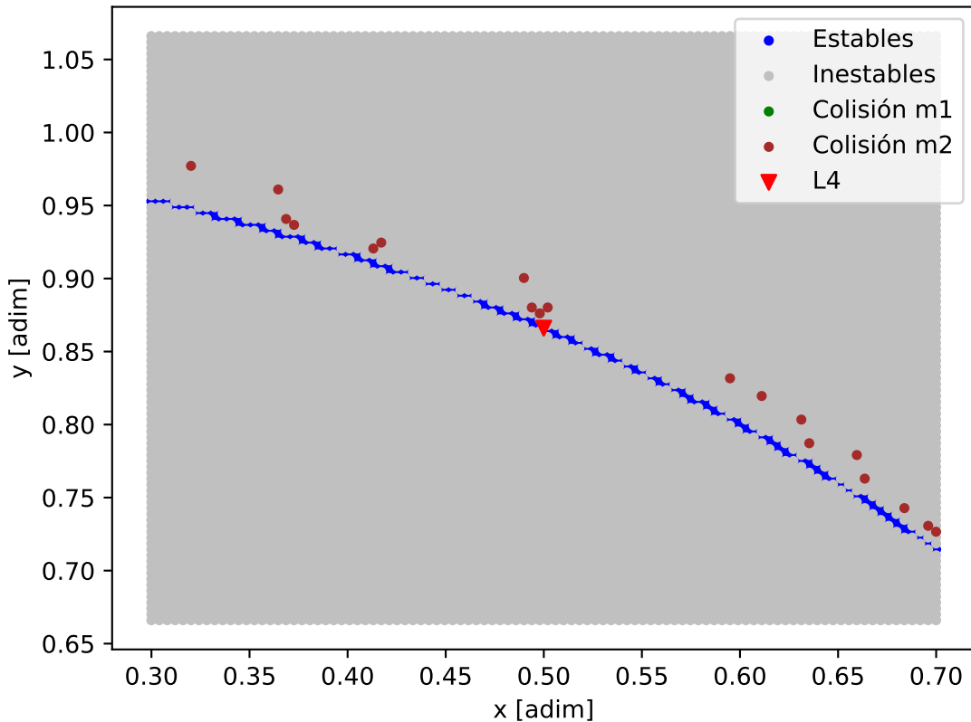
Mapa de estabilidad - HD_106315_HD_106315_b
