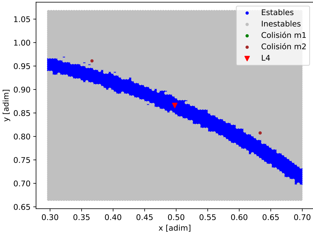
Mapa de estabilidad - HD_113337_HD_113337_b
