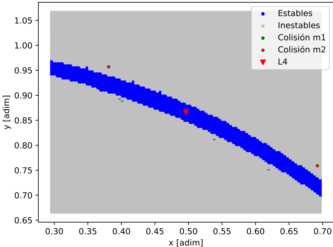
Mapa de estabilidad - HD_13908_HD_13908_c
