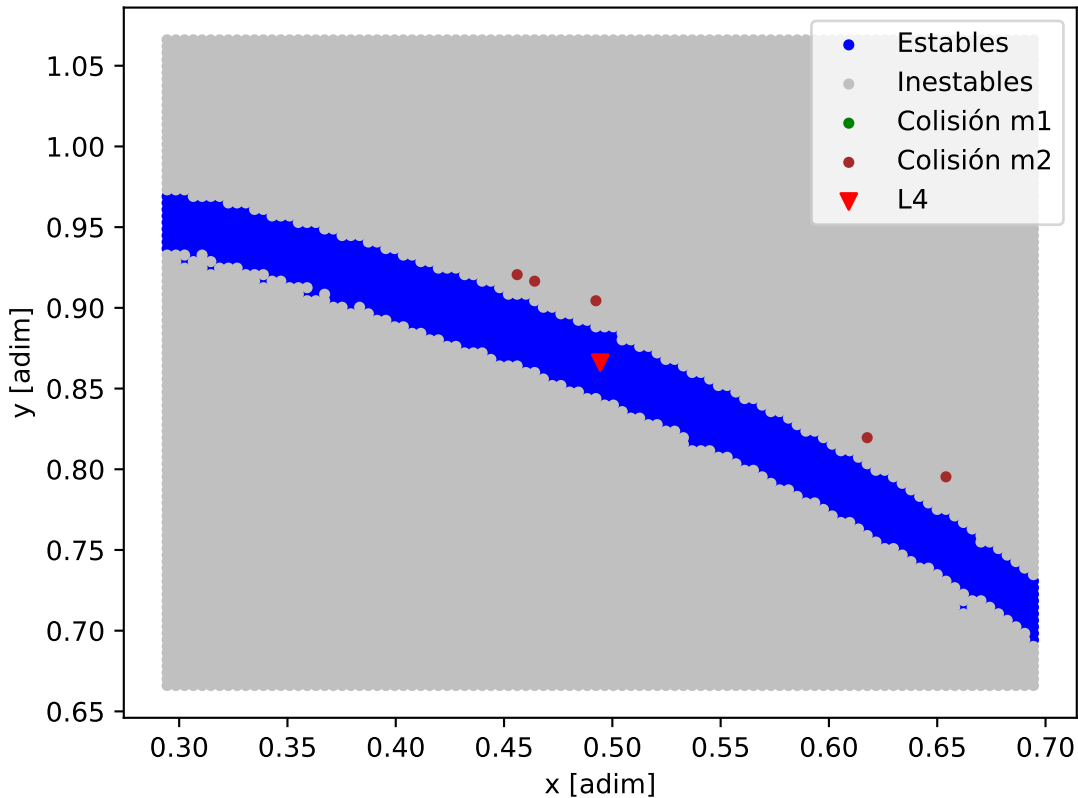
Mapa de estabilidad - HD_142_HD_142_b
